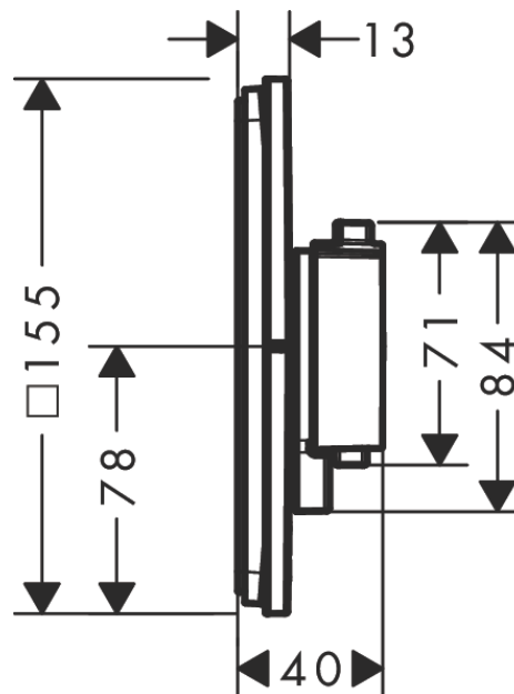
Kótovaný výkres
