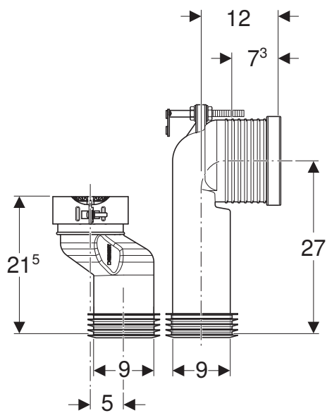
Geberit iCon TurboFlush
